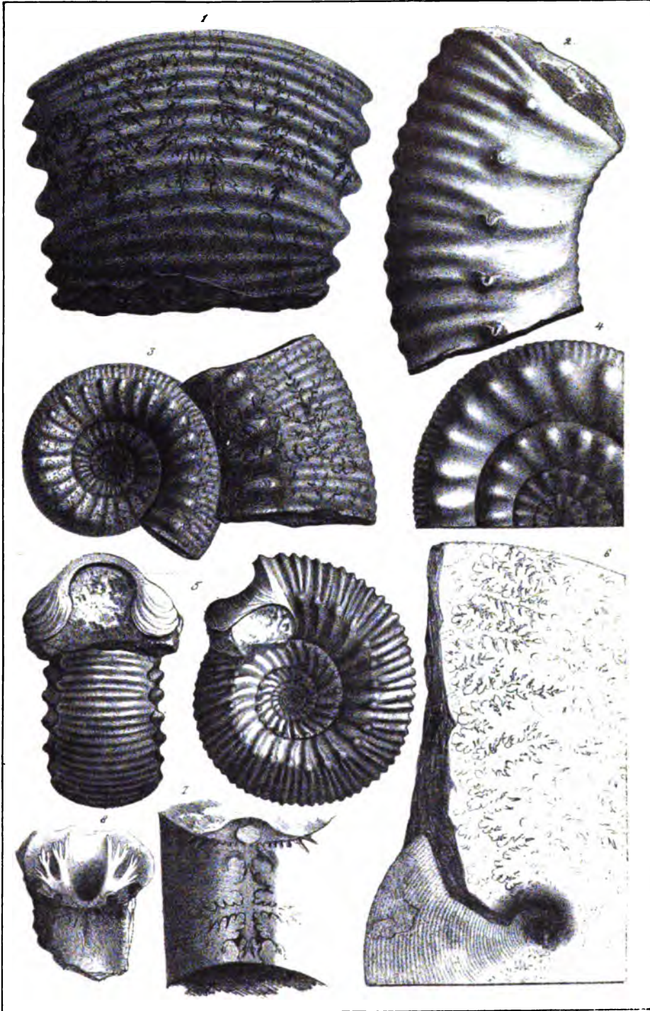
Quenstedt Jura.
